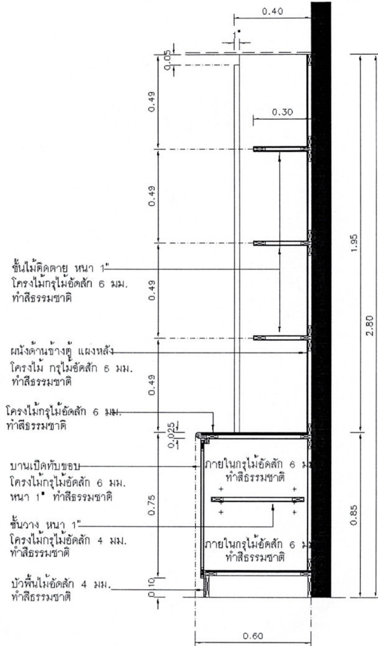
รูปตัด 1 ตู้ BUILT-IN
