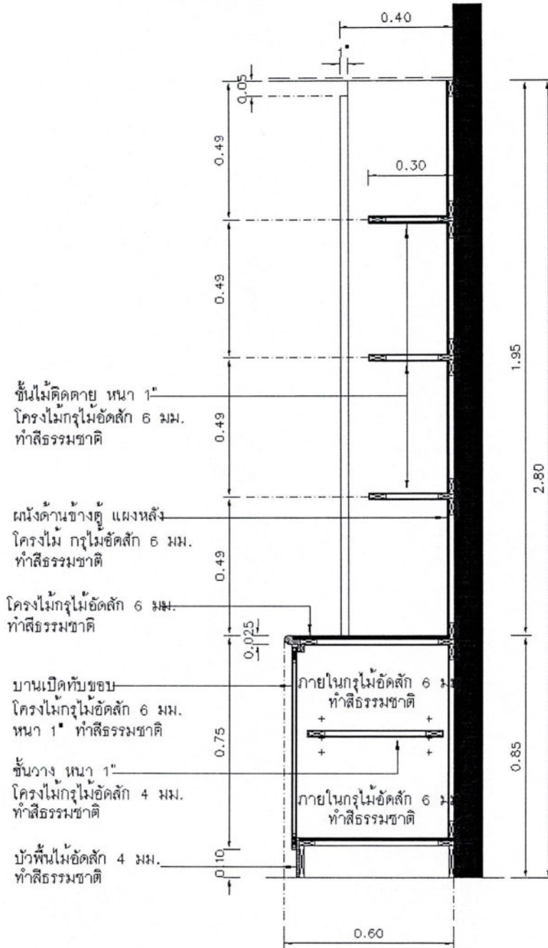
รูปตัด ตู BUILT-IN 1
