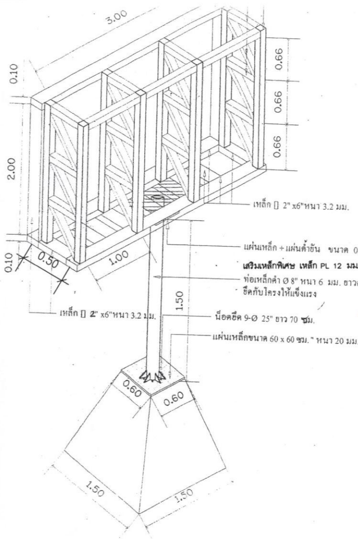
รูปขยายโครงสร้างป้าย LED มาตรฐาน 1:50
