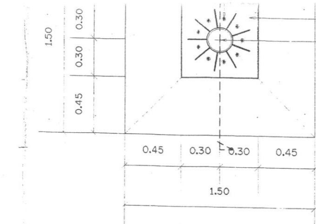
แปลนเสาป้าย LED มาตรฐาน 1:25
